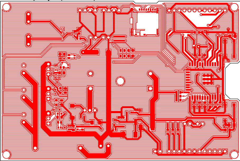
Trilhas Top Layer (Scale 1:1)
