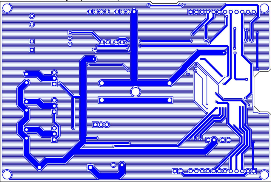
Trilhas Bottom Layer (Scale 1:1)
