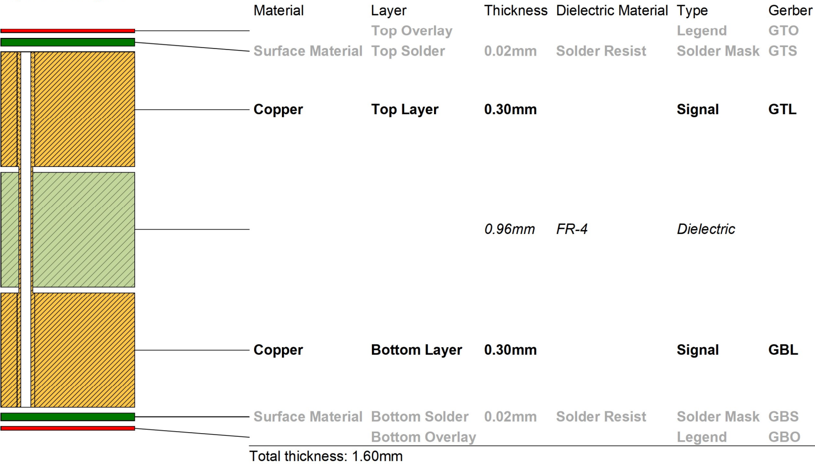
Layer Stack Legend
